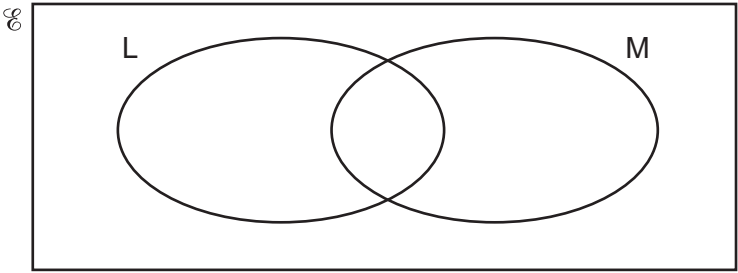
Venn diagram 1:
