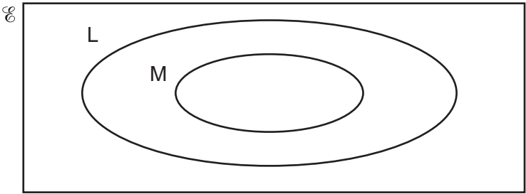
Venn diagram 3:
